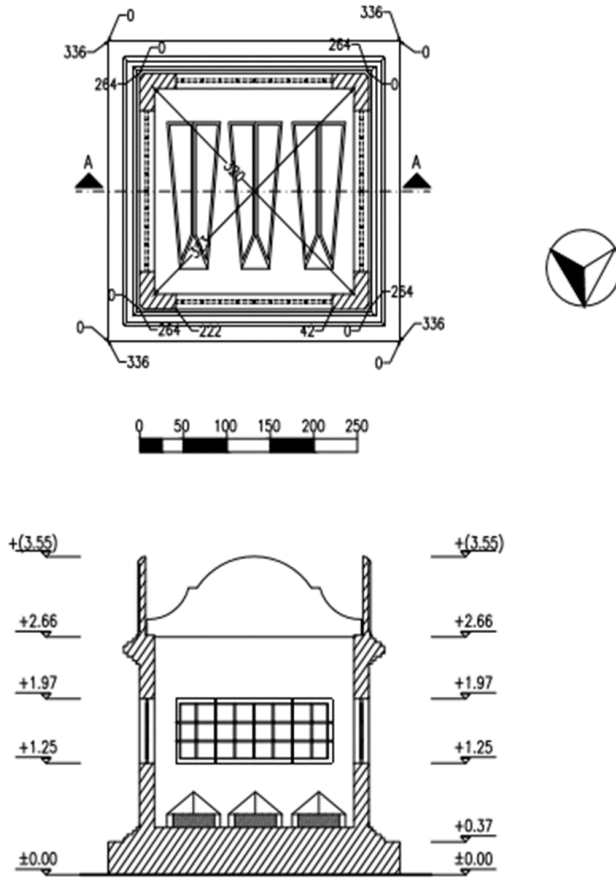
Şekil 1: Ahmed Kuddusi Mezar Anıtı röleve ve restitüsyon planı (Çizim: Humam Hamid).
